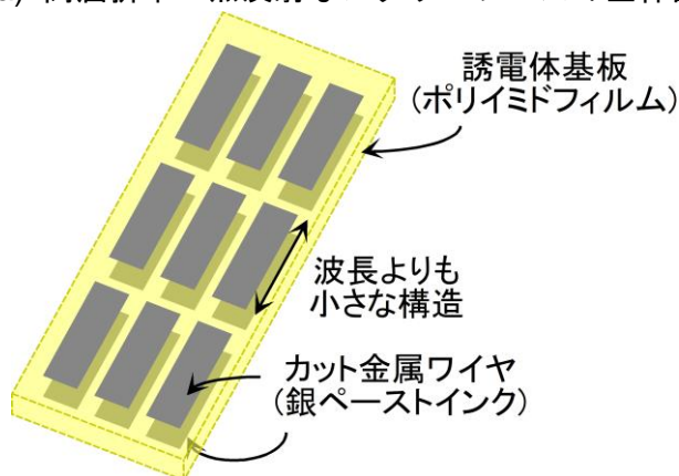
(b) カット金属ワイヤーからなるメタアトムの拡大図
