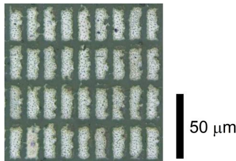
(b) カット金属ワイヤーからなるメタアトムの大写真
